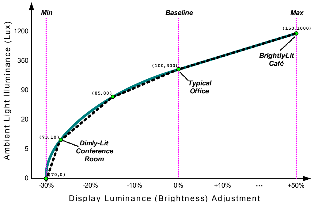
Figure 9-51 A five-point ALS Response Curve
